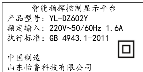
产品铭牌样式
